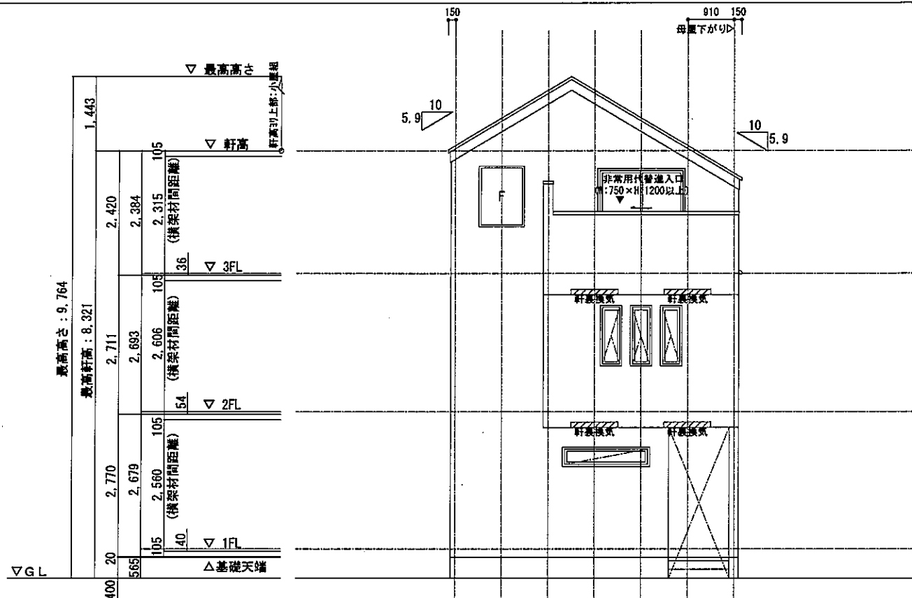
南立面图 1/100
