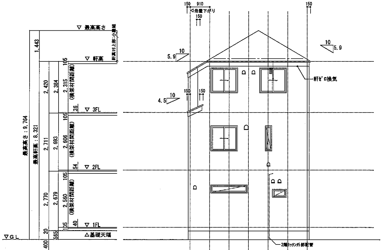
北立面图 1/100
