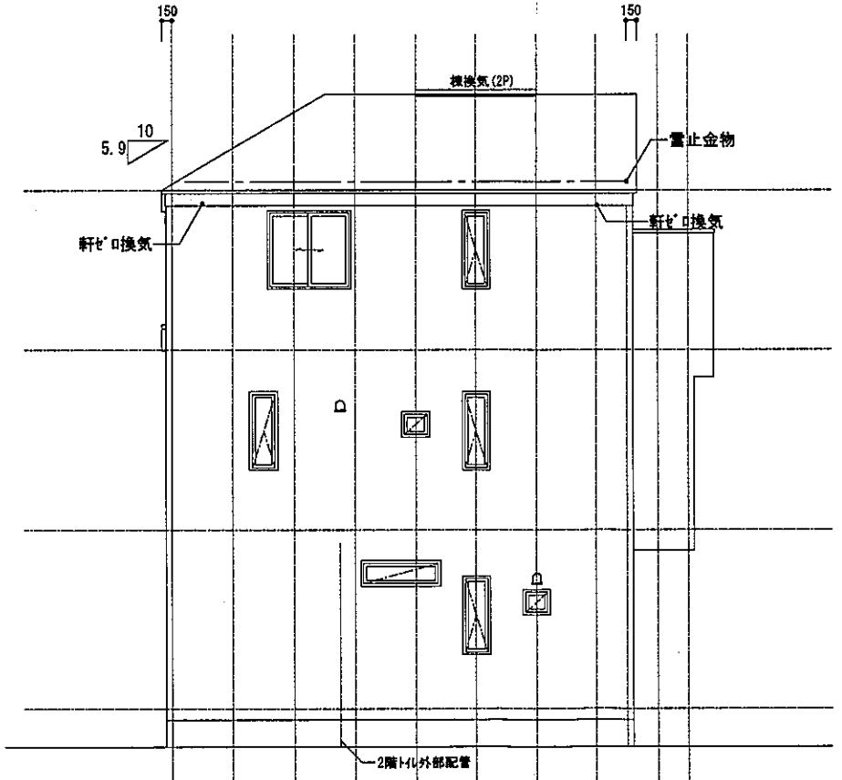
西立面图 1/100
