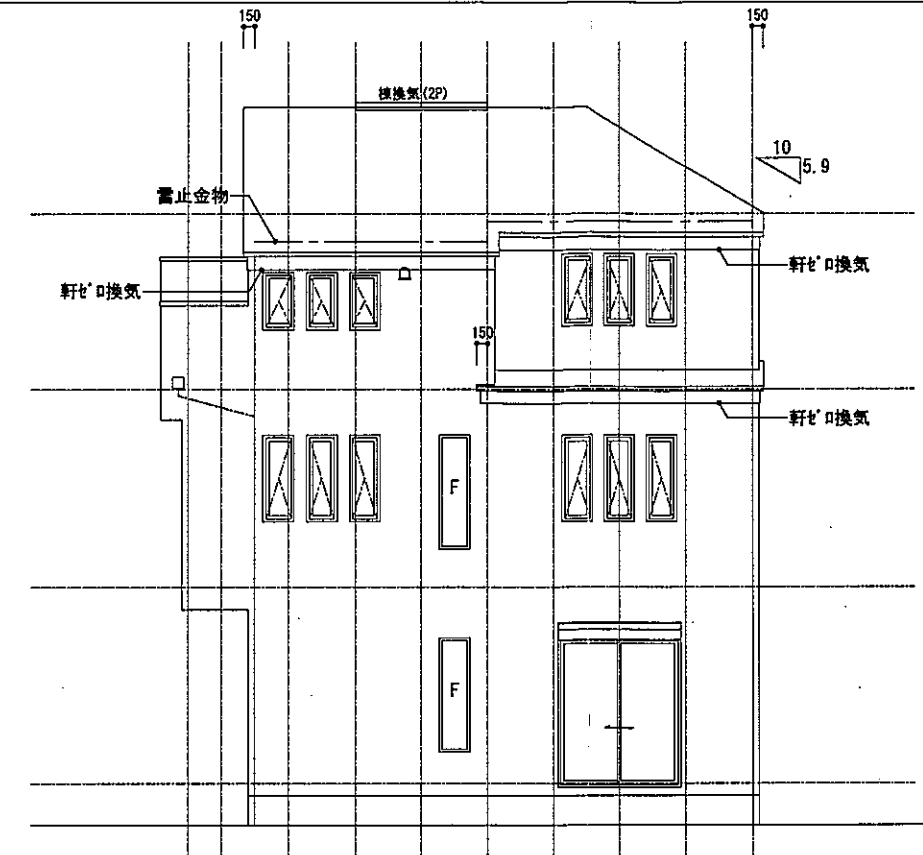
東立面图 1/100
